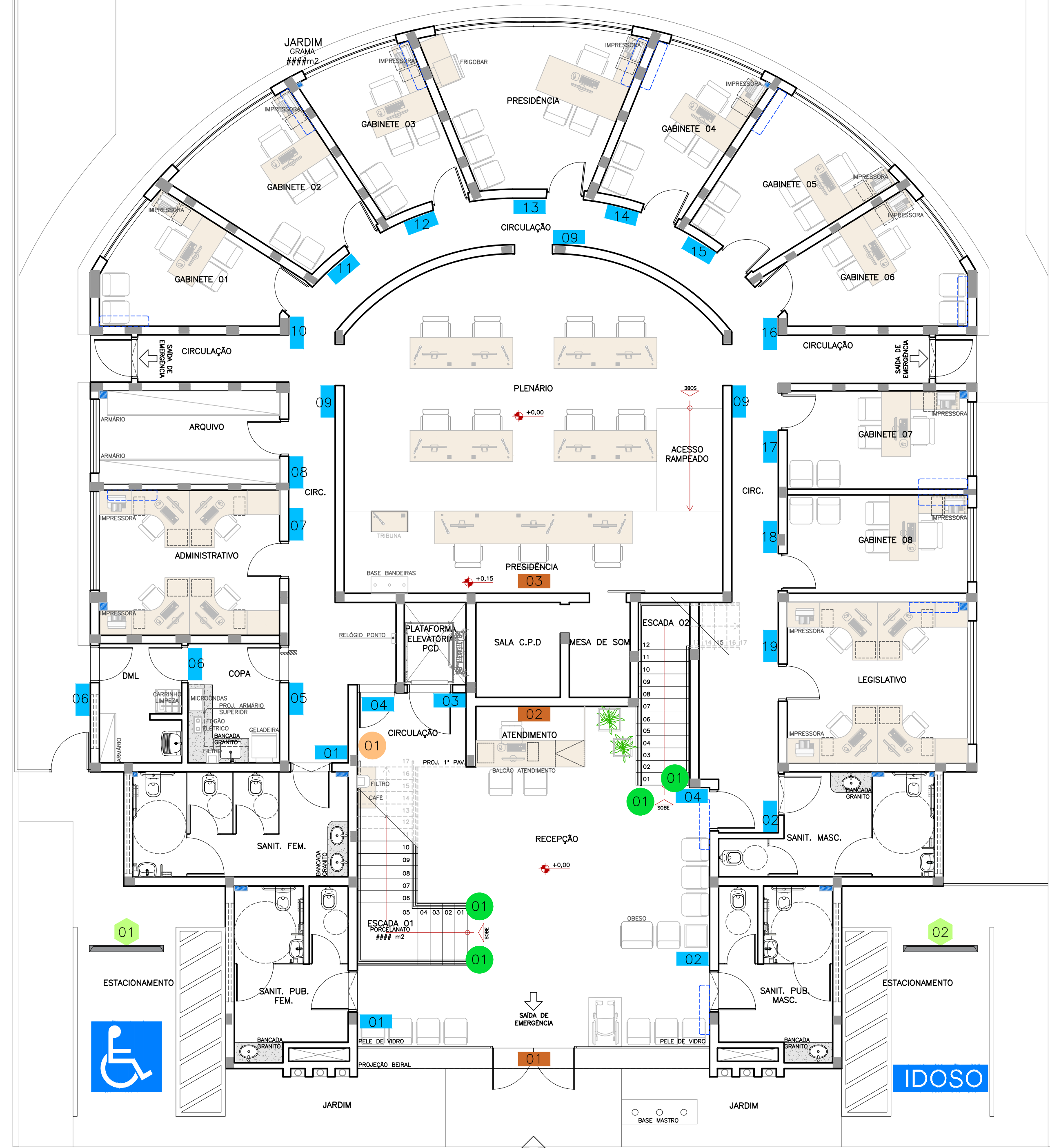
Planta Baixa - Pav. Térreo Esc.: 1/75
