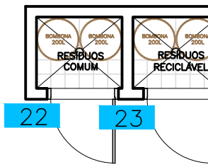
Planta Baixa - Central de Resíduos Esc.: 1/75
