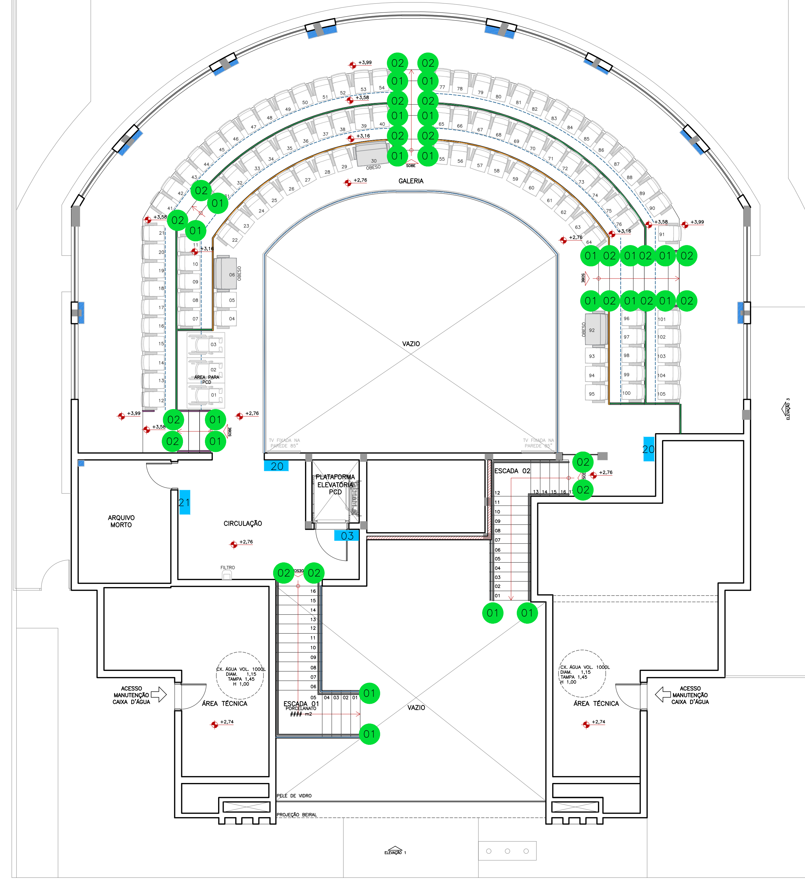
Planta Baixa - Pav. Superior Esc.: 1/75
