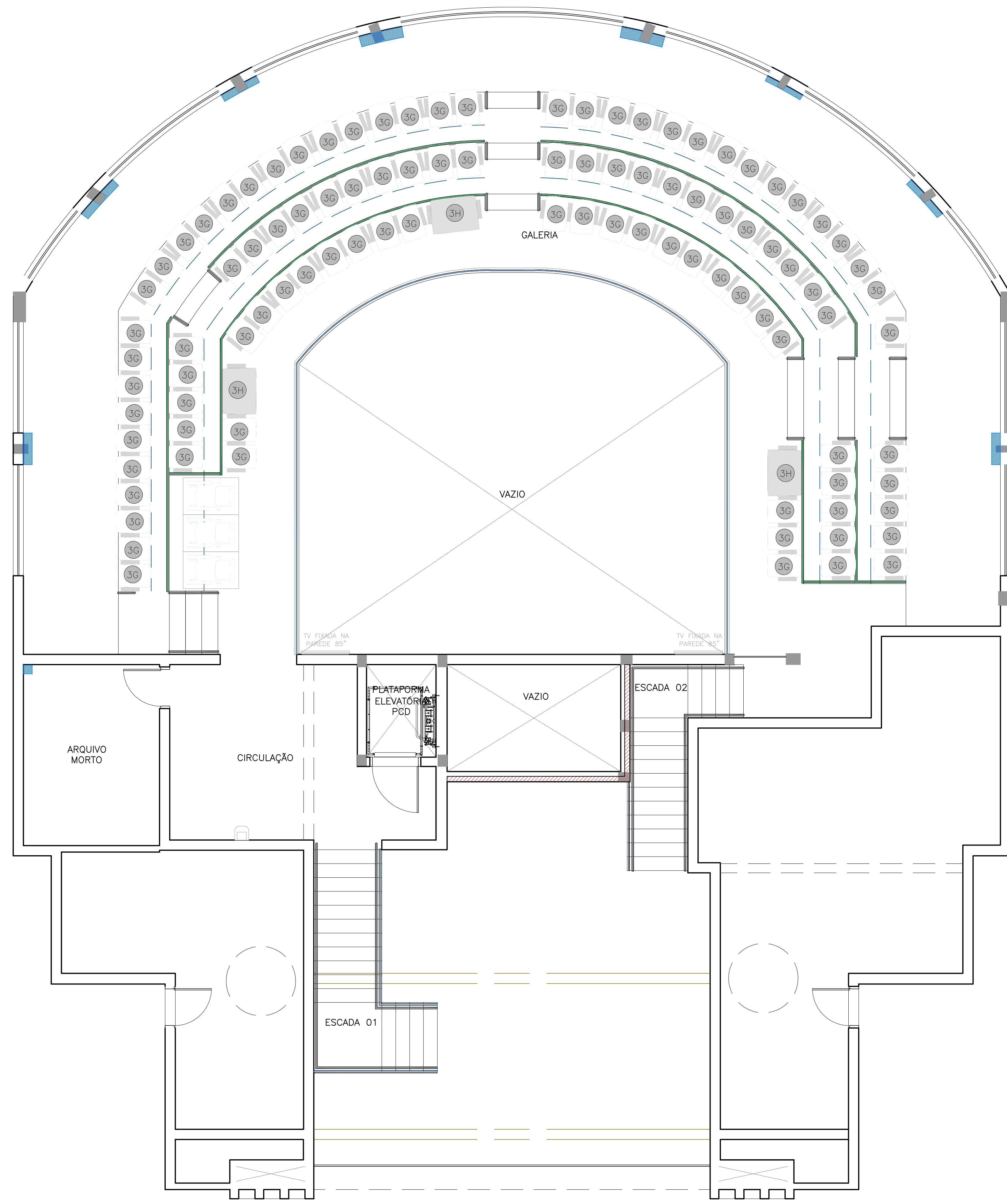
Planta Baixa - Mobiliário Planimetria: Tamo Esc.: 1:50
