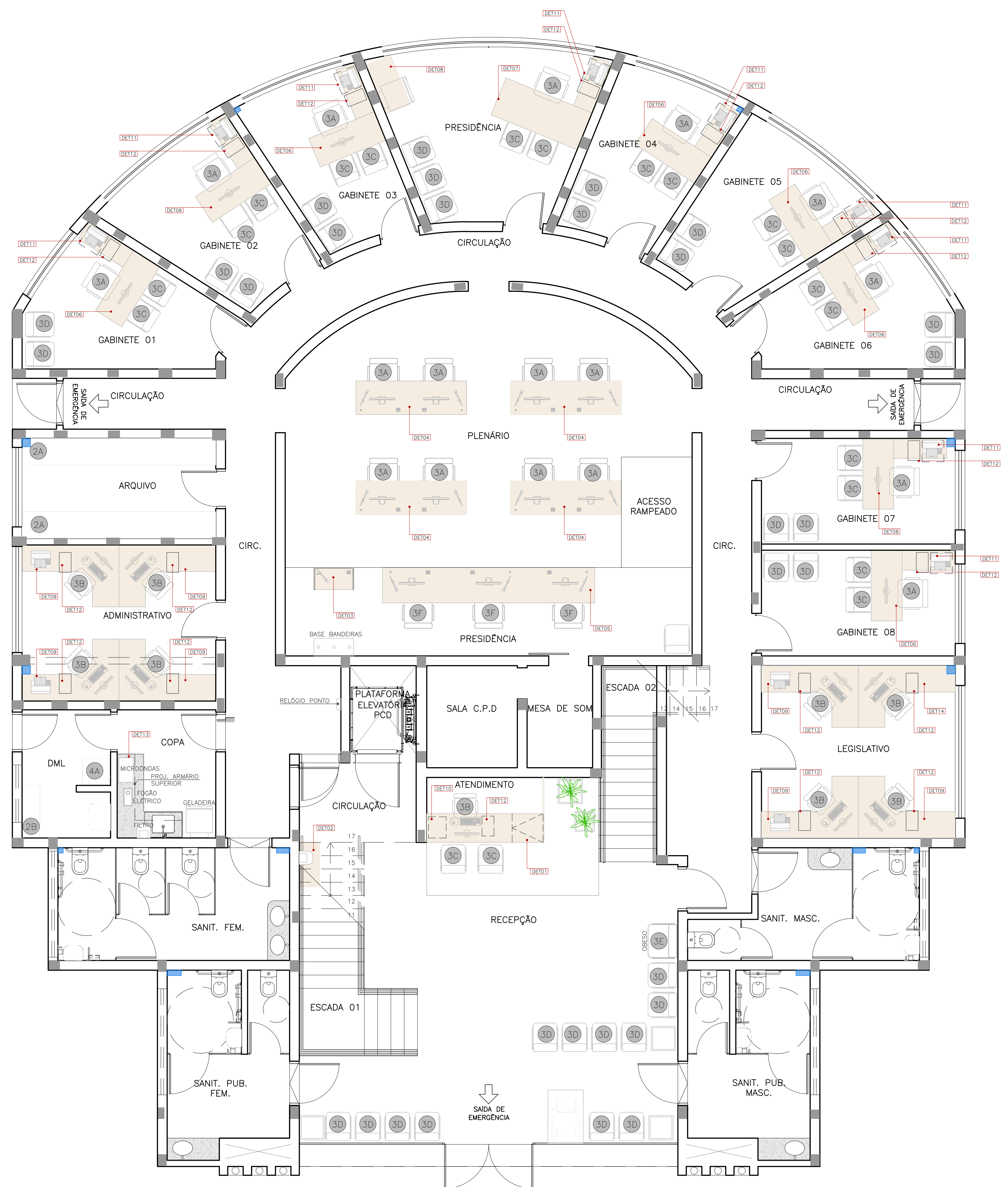
Planta Baixa - Mobiliário Planimetria: Tamo Esc.: 1:50
