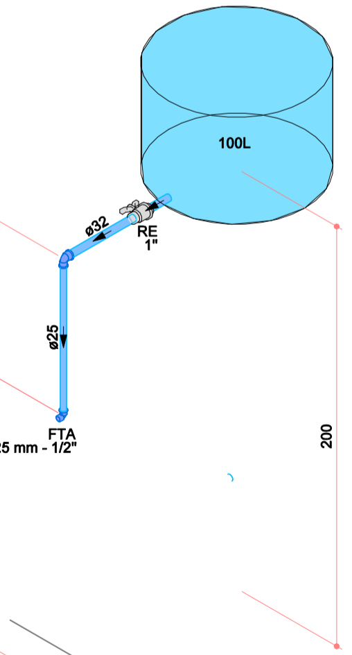
Detalhe HID-4 Escala 1:25
