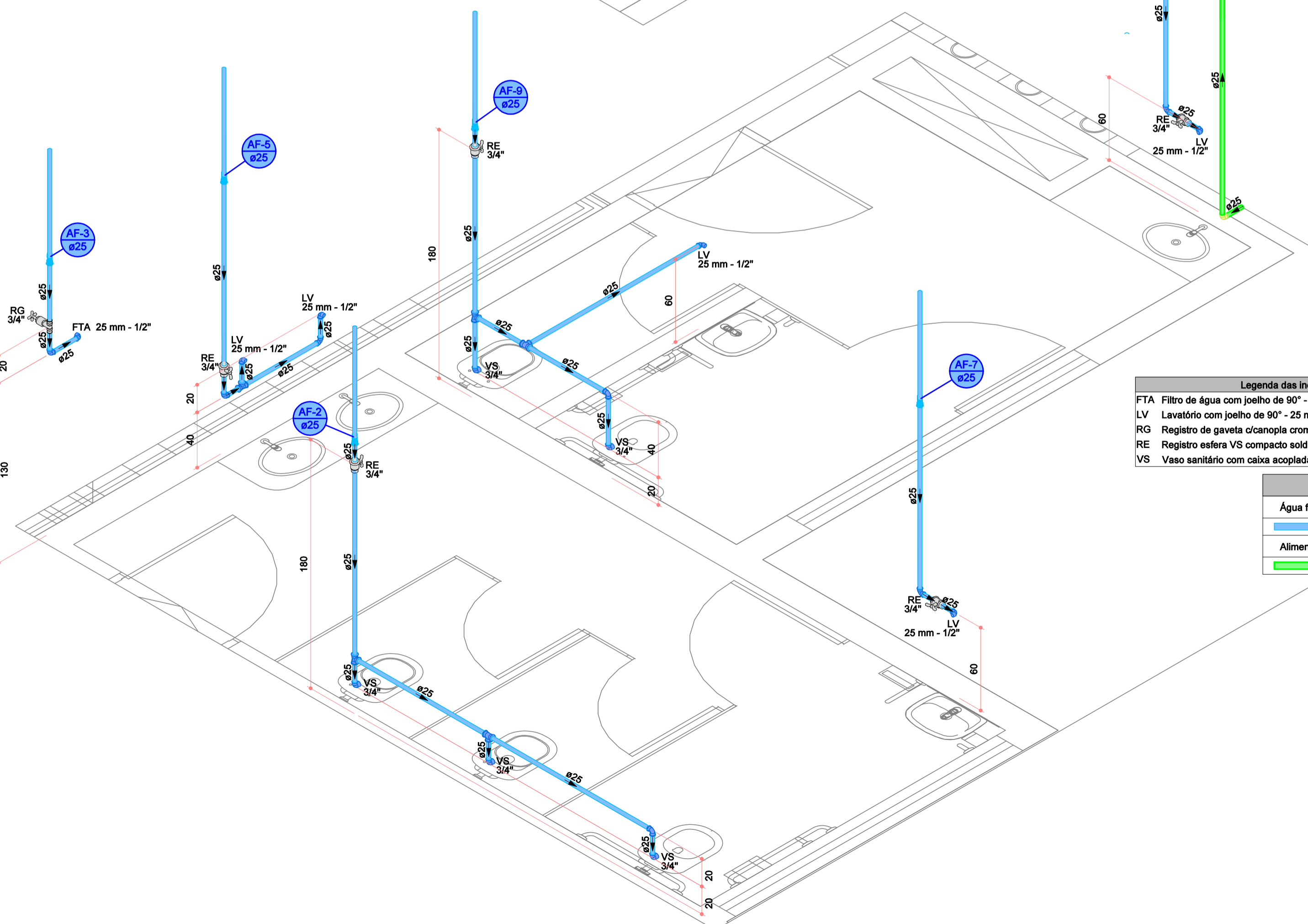
Detalhe HID-3 Escala 1:25
