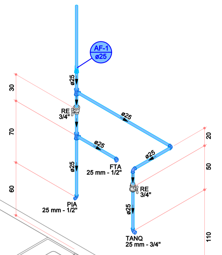
Detalhe HID-1 Escala 1:25
